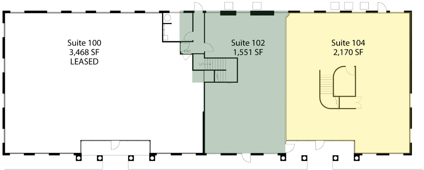
01 LEVEL 1 SCALE: 1/8" = 1'-0"
